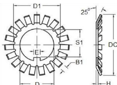
Dimensions of Metric DIN 5406 Shaft Tab Washer
